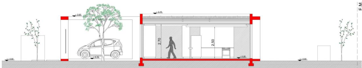
Corte Longitudinal
