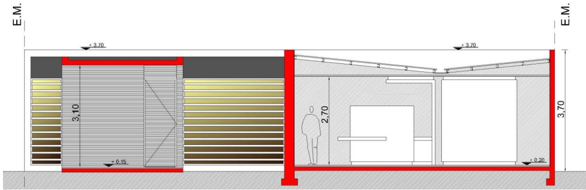
Corte Transversal
